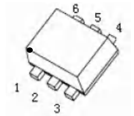
SOT-563
